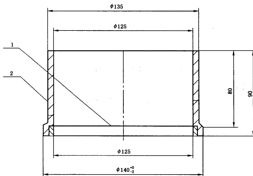
图 2 水筛
