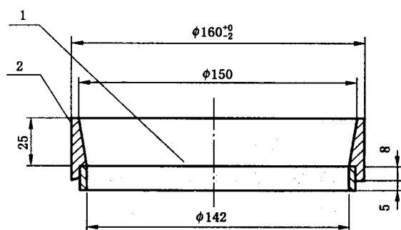
图 1 负压筛
