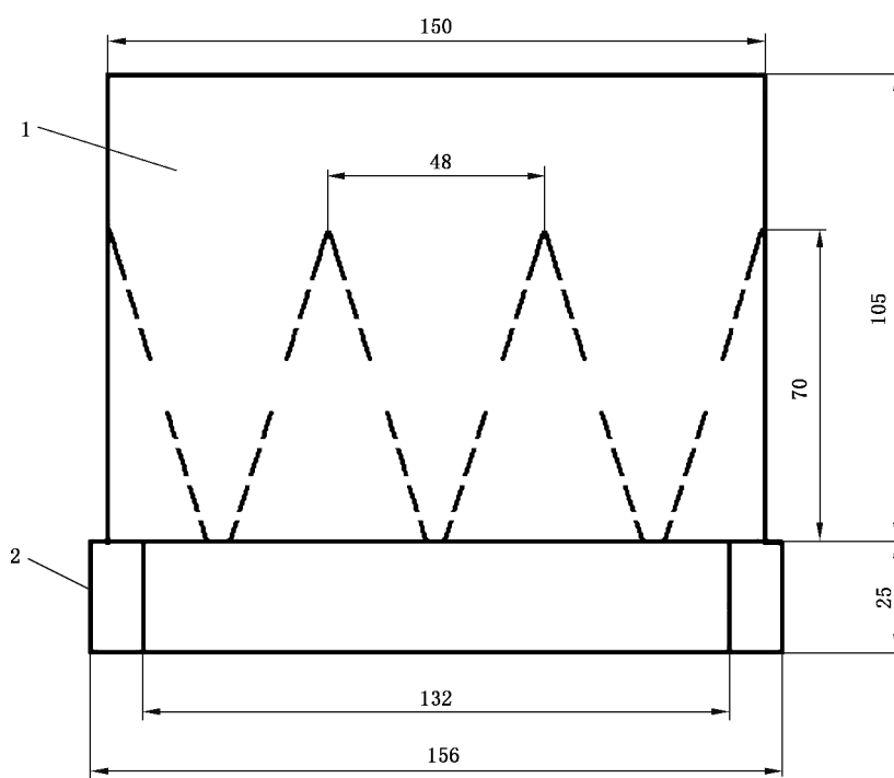
图 5 胶砂振动台示意图
